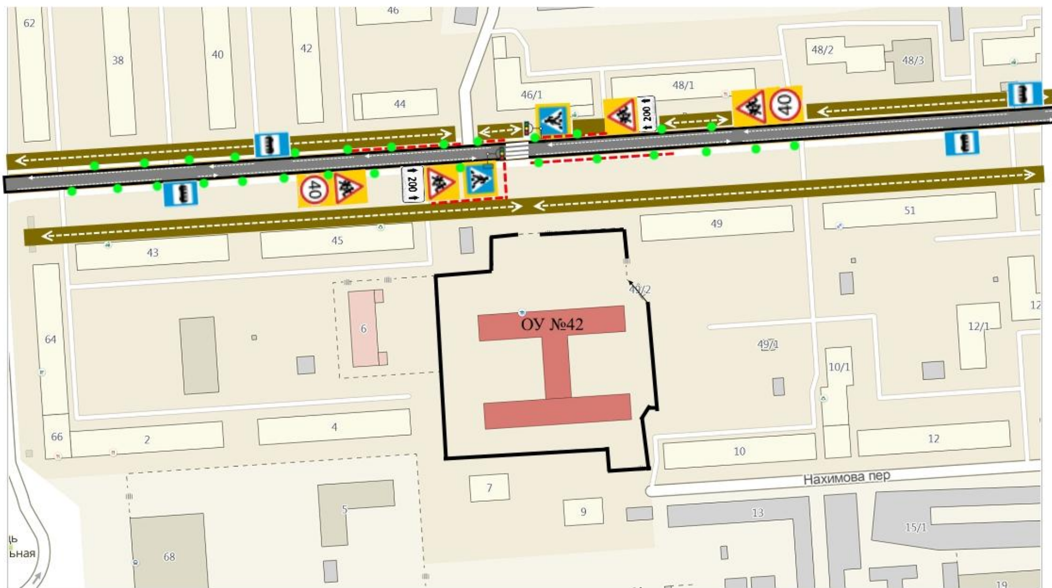
План-схема организации дорожного движения в непосредственной близости от МОУ СОШ № 42 с размещением соответствующих технических средств, маршруты движения обучающихся и расположение парковочных мест.
